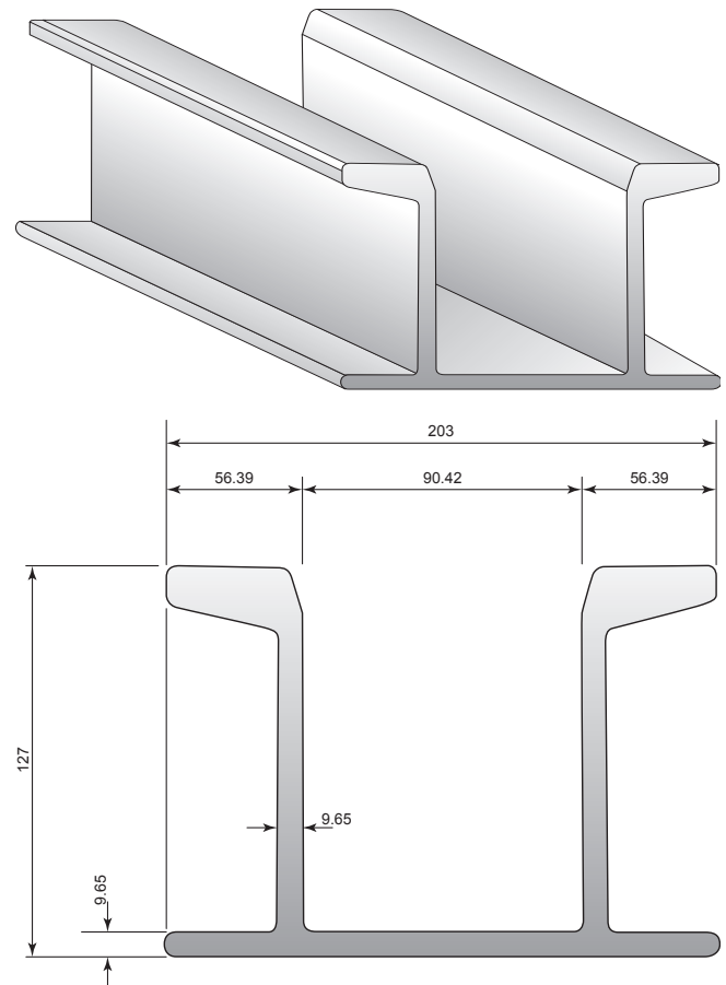
Coupe transversale du rail résistant de Waler Dimensions en Millimètres (mm)
